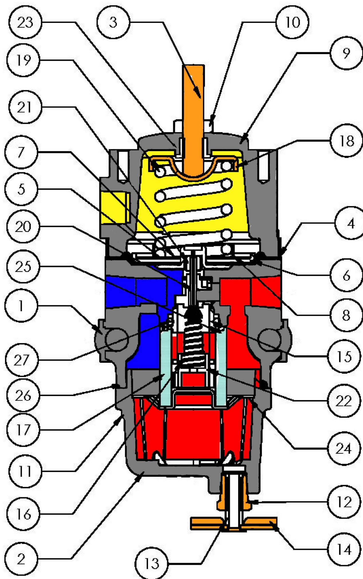
Despiece de filtro regulador.
